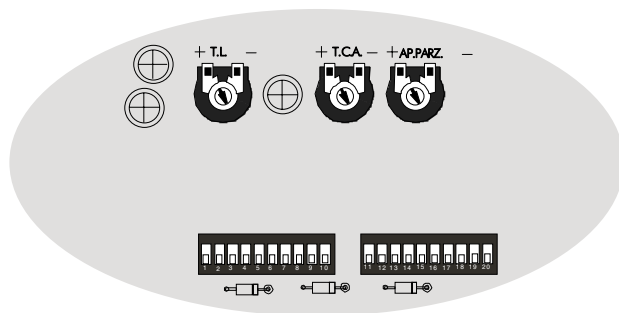
Scheda base del motore "A" "A" Motor main board Carte de base du moteur "A" Basiskarte vom Motor "A" Tarjeta base del motor «A»
