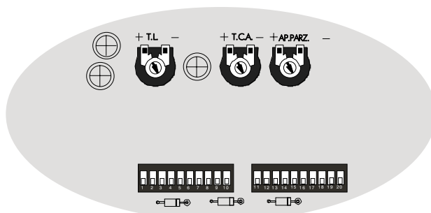
Scheda base del motore "B" "B" Motor main board Carte de base du moteur "B" Basiskarte vom Motor "B" Tarjeta base del motor «B»
