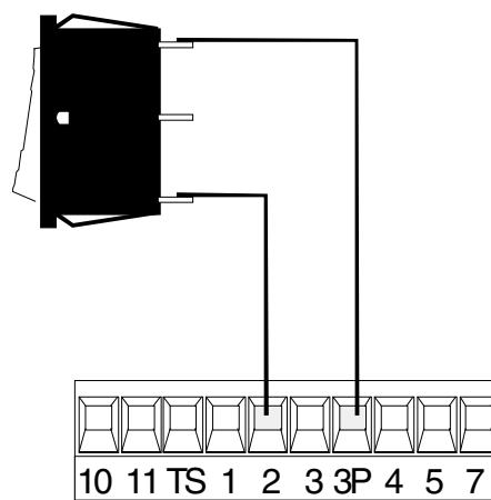
Pulsante (N.O.) «Apertura parziale» «Partial opening» button (N.O.) Bouton-poussoir (N.O.) «Ouverture partial» Taste (Arbeitskontakt) «Teilöffnung» Pulsador (N.O.) «Apertura parcial»
